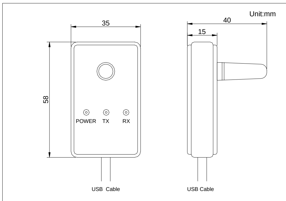
6.外形尺寸结构示意图（下图,单位：毫米）：
